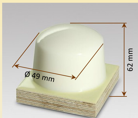
Druckbild/Image: Ø ca. 35 mm Nr./No.: 2014
