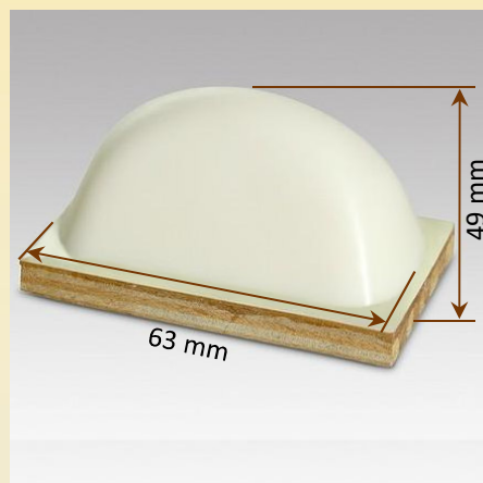
Druckbild/Image: ca. 10 x 50 mm Nr./No.: 3009
