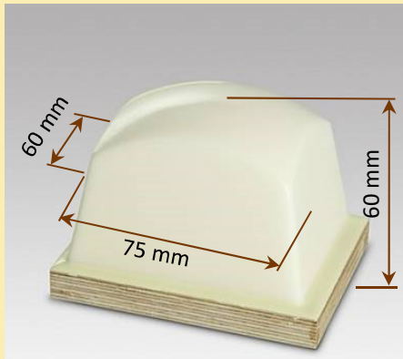
Druckbild/Image: ca.45x60mm Best.-Nr.: 2041
