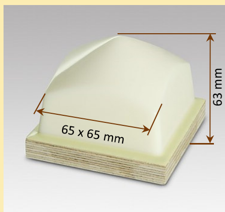
Druckbild/Image ca. 45 x 45 mm Nr./No.: 2061
