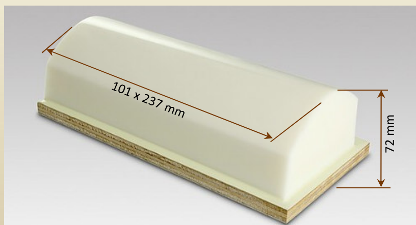
Druckbild/Image: ca. 75 x 200 mm Nr./No.: 4002
